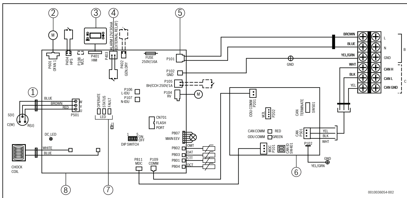
26. ábra Kapcsolási rajz – kültéri egység, egy fázis, CS3400iAWS 4 OR-S
