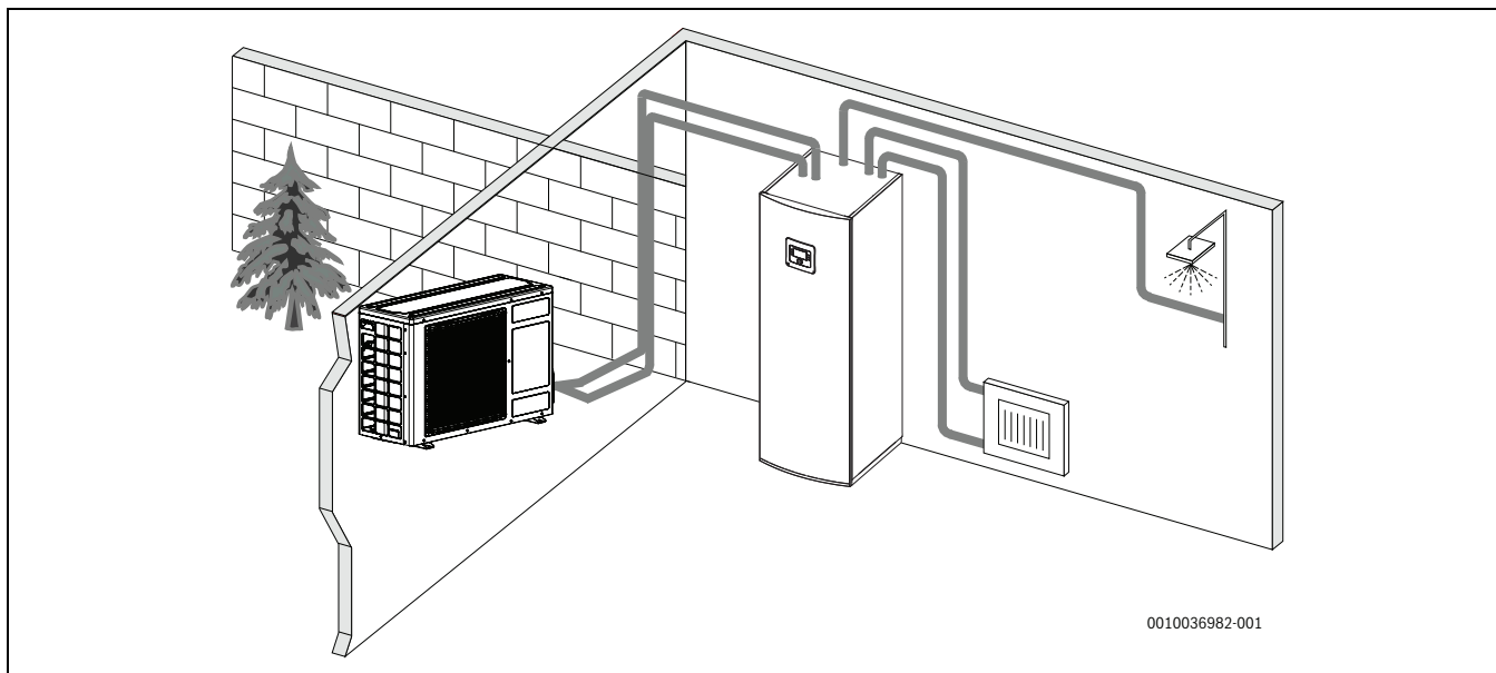
2. ábra Hőszivattyú kültéri egységhez, valamint beépített melegvíz-tárolóval és elektromos fűtést segítővel rendelkező AWS M beltéri egységhez
