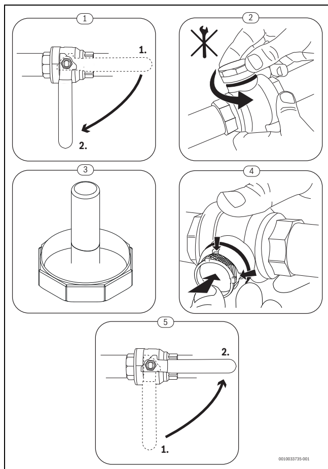
5. ábra A szűrő tisztítása
