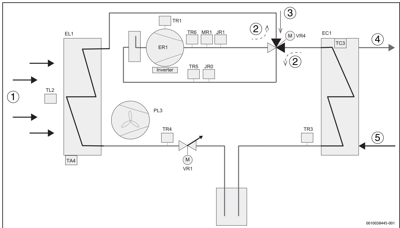
48. ábra Hűtőközegkör
