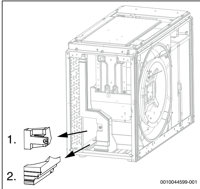
44. ábra EPP alkatrészek
