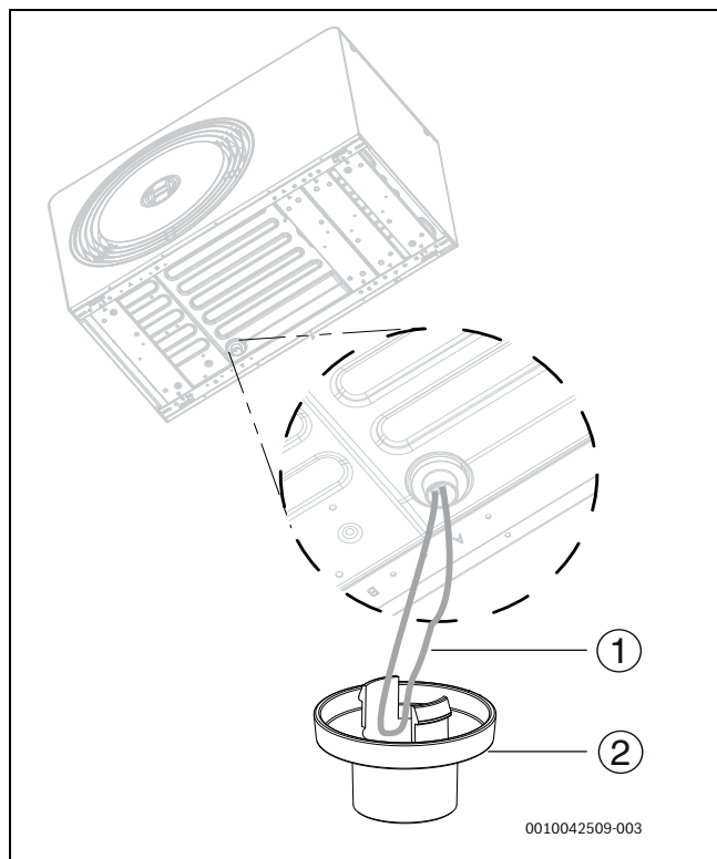
28. ábra A lefolyóvezeték-csatlakozó szerelése
