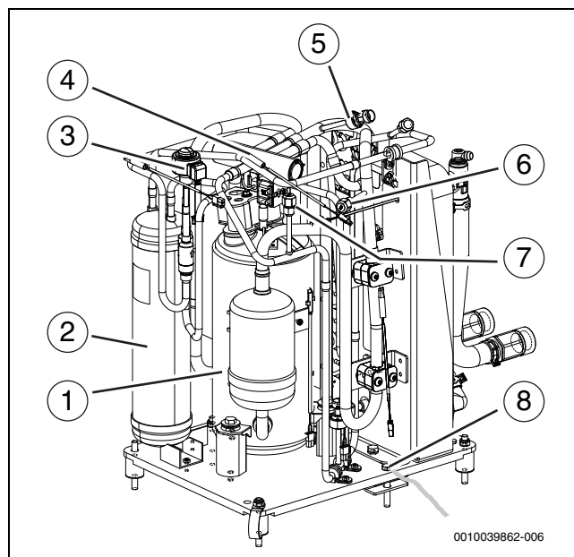
2. ábra Termékáttekintés – előlnézet
