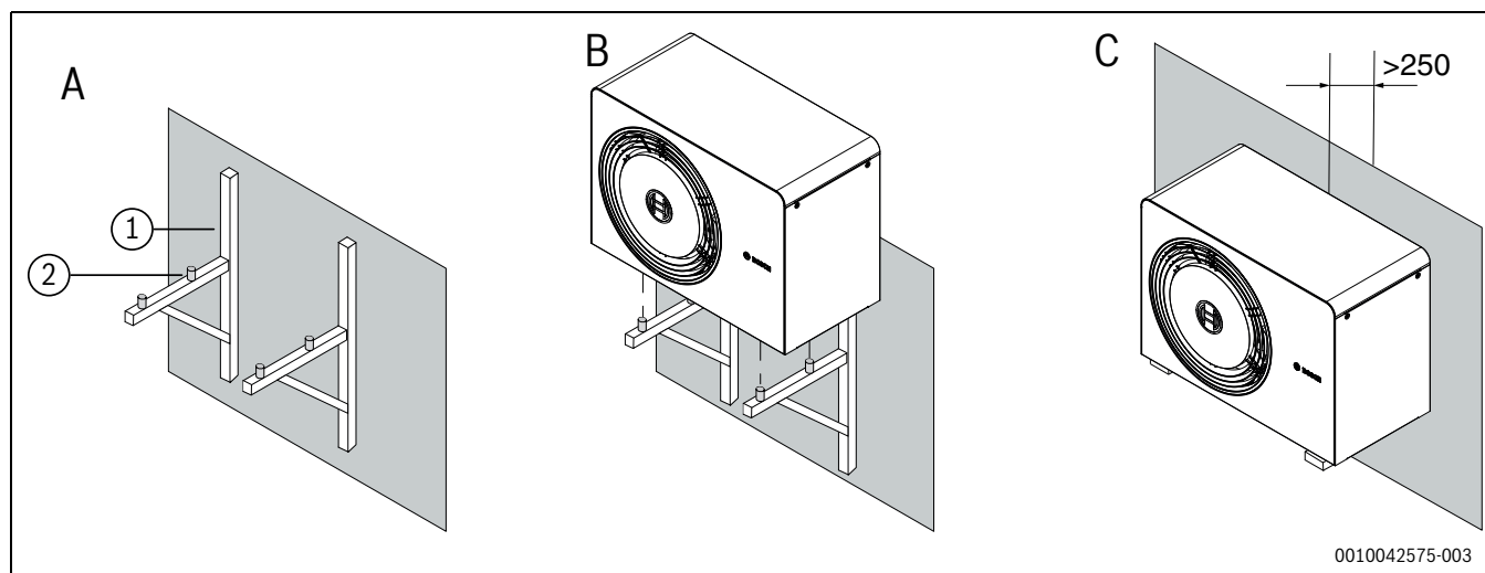
26. ábra Falra szerelt kültéri egység (mm)
