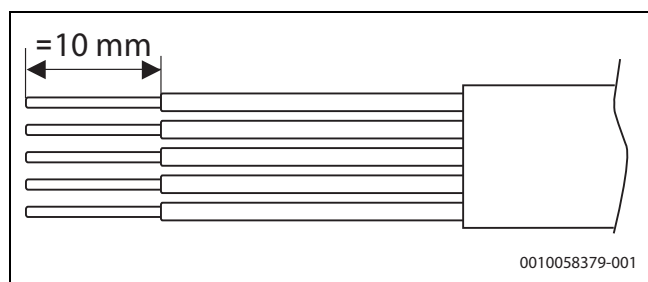
41. ábra Kábelblankolás a tápellátási csatlakozókábelek esetében
