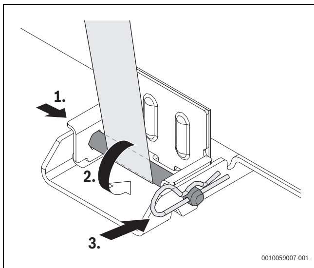
14. ábra A rögzítőkonzol, a csap és a heveder behelyezése
