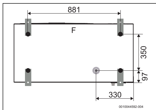
6. ábra Távolságok a leeresztő csonttól – alulnézet
