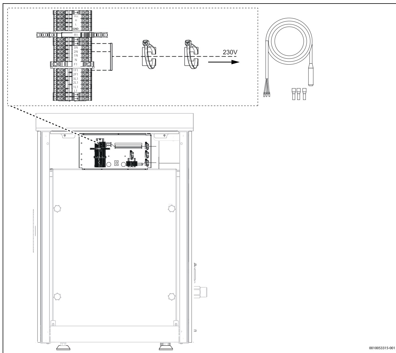
42. ábra A fűtőkábel csatlakoztatása (külön rendelhető tartozék)
