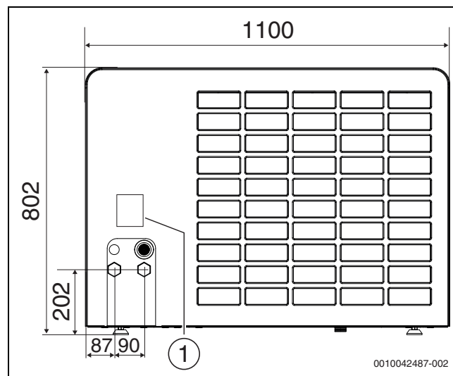
4. ábra A hőszivattyú méretei és csatlakozásai – hátulnézet
