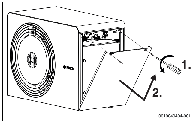
34. ábra Oldalsó burkolat
