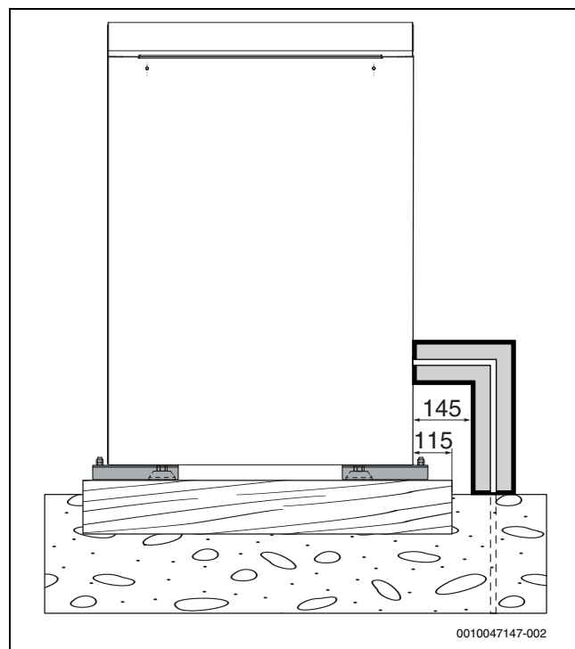
24. ábra Oldalnézet szerelőkészlettel
