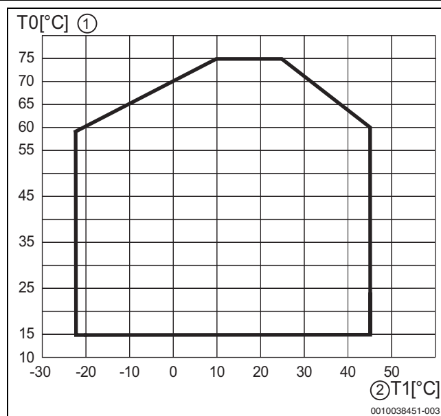
46. ábra Hőszivattyú fűtési üzemben elektromos fűtőbetét nélkül
