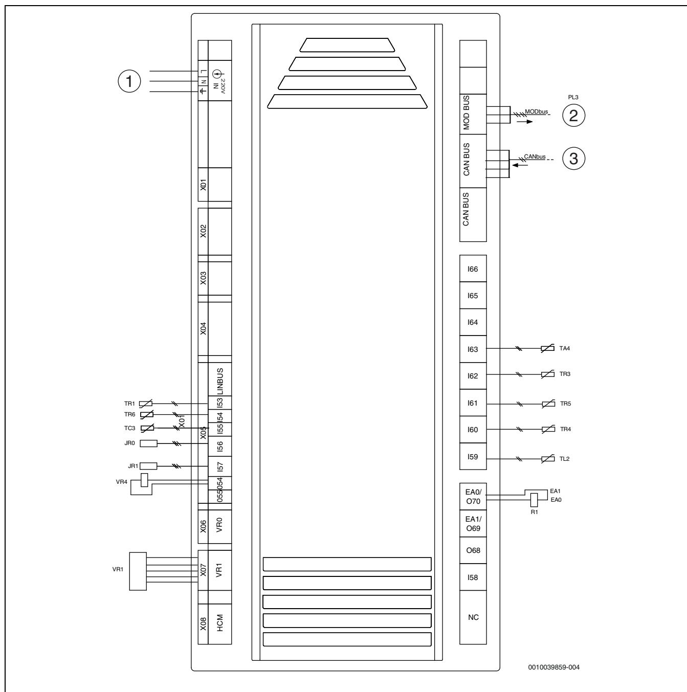
50. ábra Kapcsolási rajz XCU-SRH (XCU-HP)
