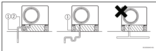
30. ábra Kondenzvízkifolyó a csatornarendszerbe / esővíz-elvezetőbe
