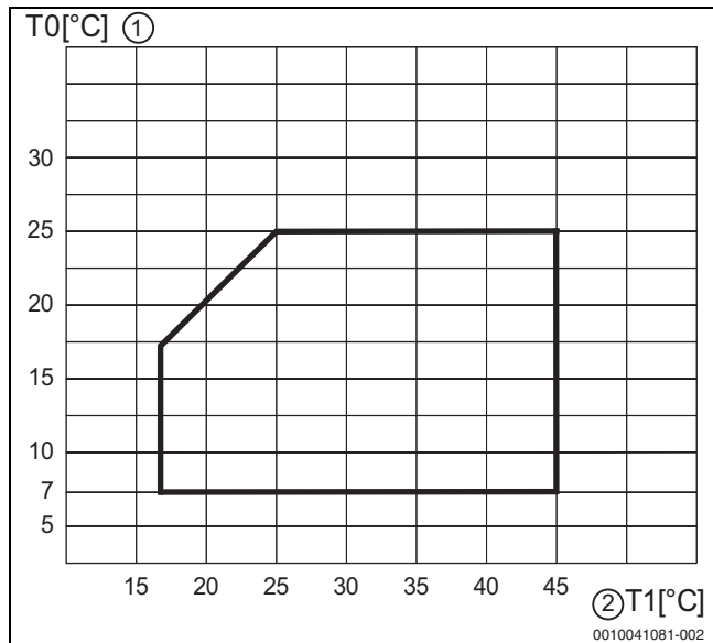
47. ábra Hőszivattyú hűtési üzemben
