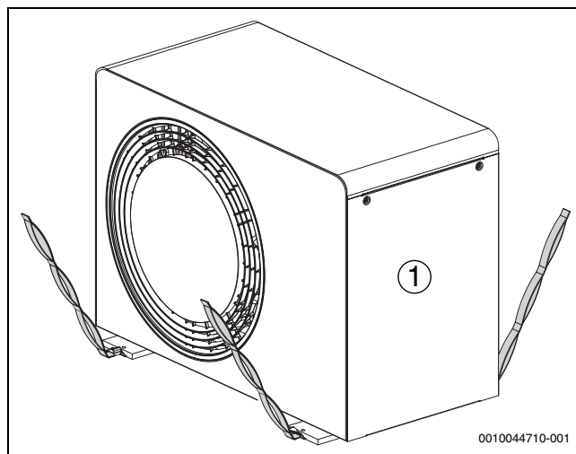
12. ábra Hevederek használata a hőszivattyú csomagolás nélküli szállításakor
