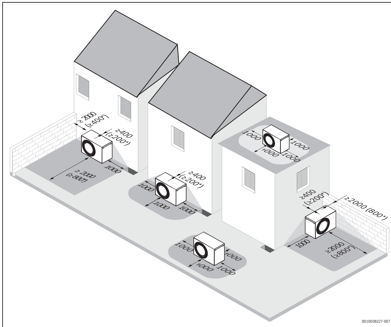
19. ábra Ajánlott távolság a hőszivattyú és a környező rögzített tárgyak között (mm)
