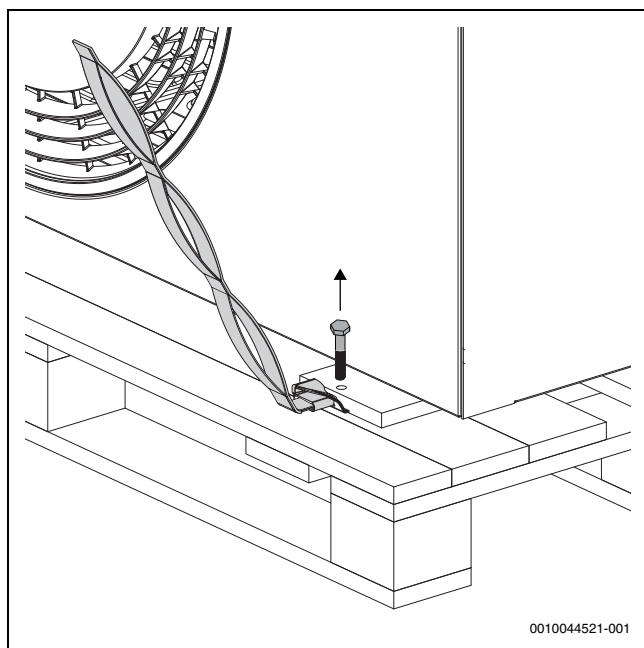
11. ábra A hevederek csatlakoztatása és a csavarok eltávolítása
