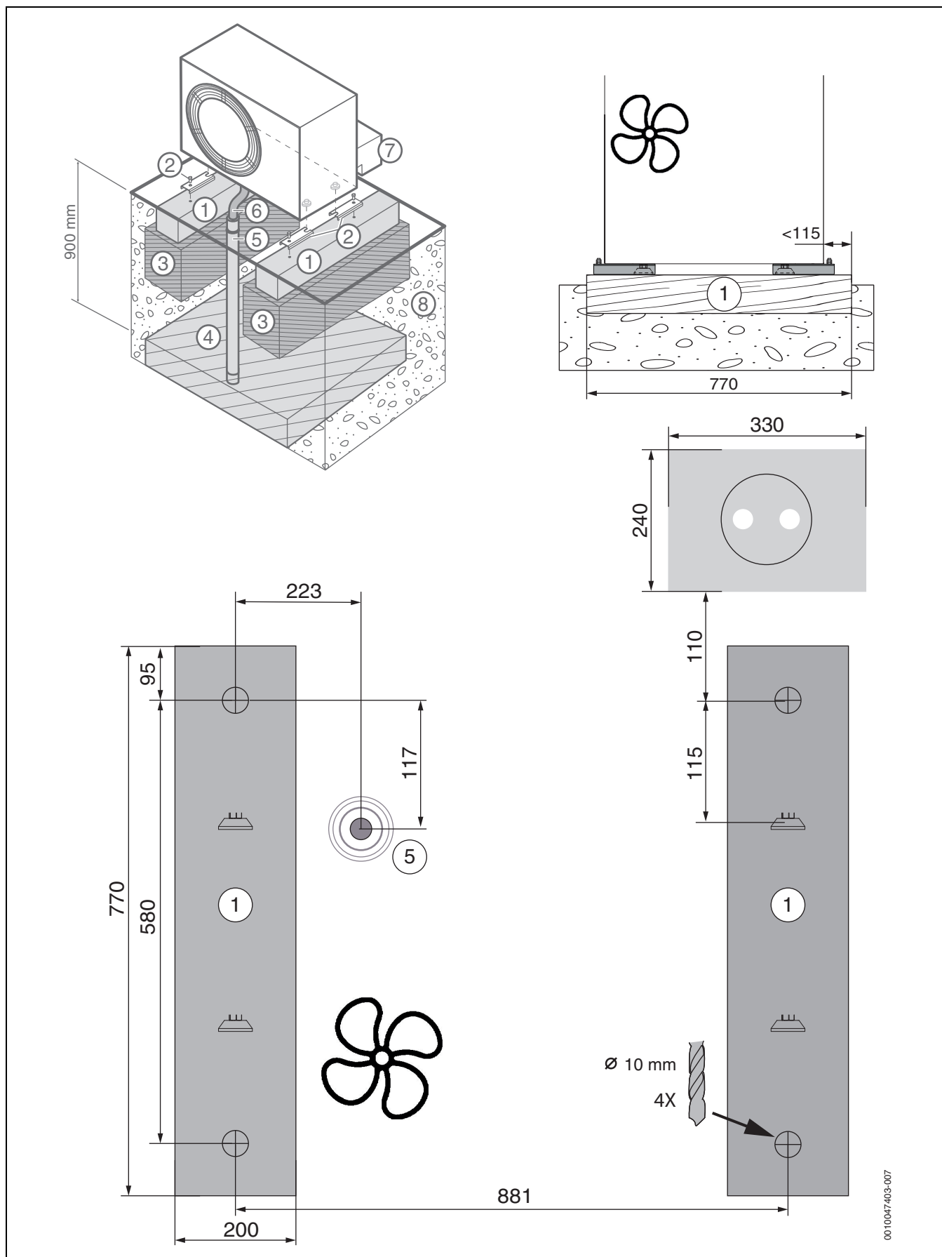
31. ábra Alapozási terv, 1. változat
