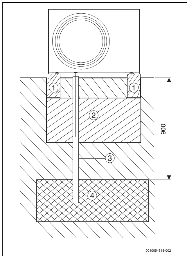
29. ábra Kondenzvíz elvezetése kavicságyba (mérték mm-ben)
