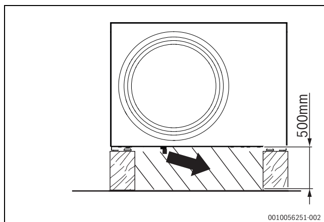
27. ábra A csepptálca fűtőkábelének szerelése
