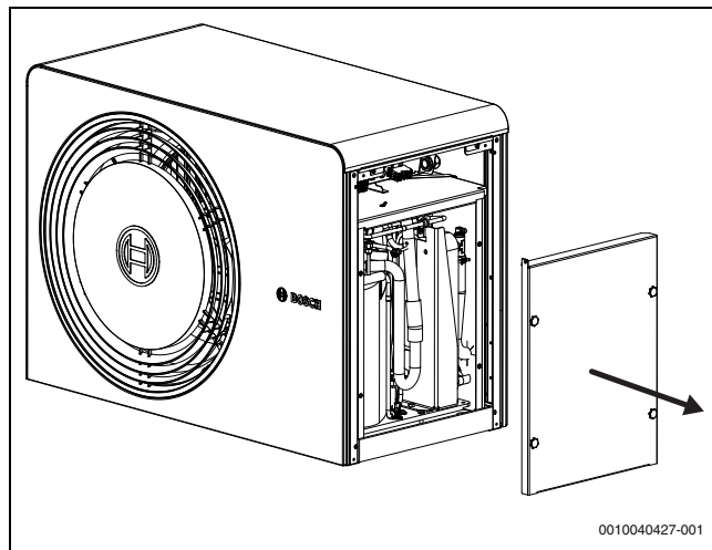
35. ábra Hűtőközegdoboz-burkolat
