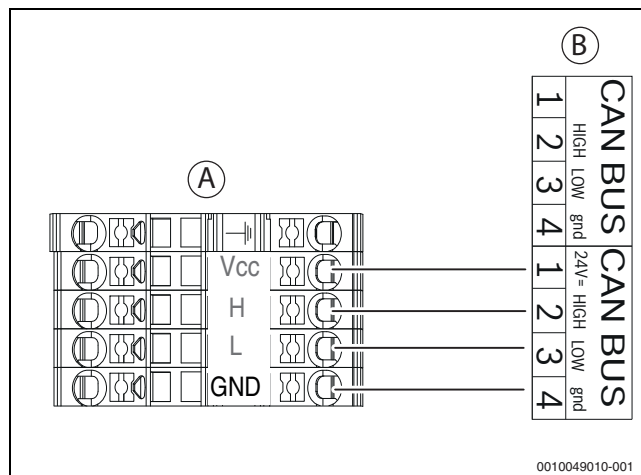
37. ábra CAN-BUS hőszivattyú – beltéri egység
