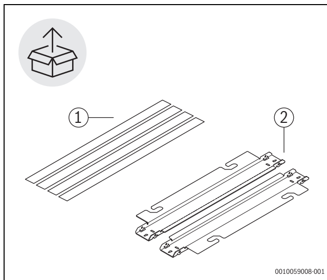
16. ábra Fém konzolok és hevederek
