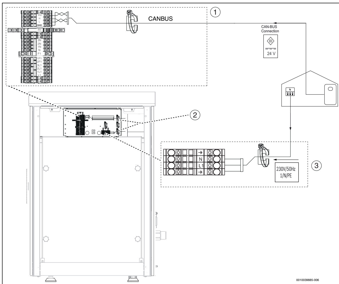
40. ábra Kapocsszekrény
