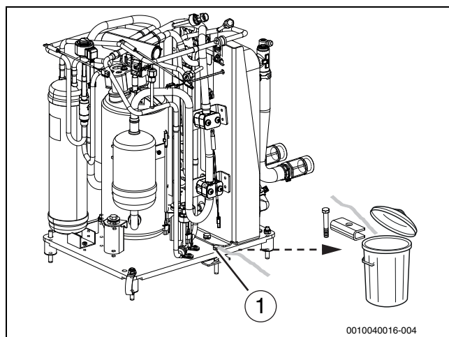
36. ábra Szállításkor alkalmazott csavar
