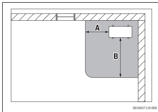
10. ábra Védőzóna talajon, sarokban elhelyezve
