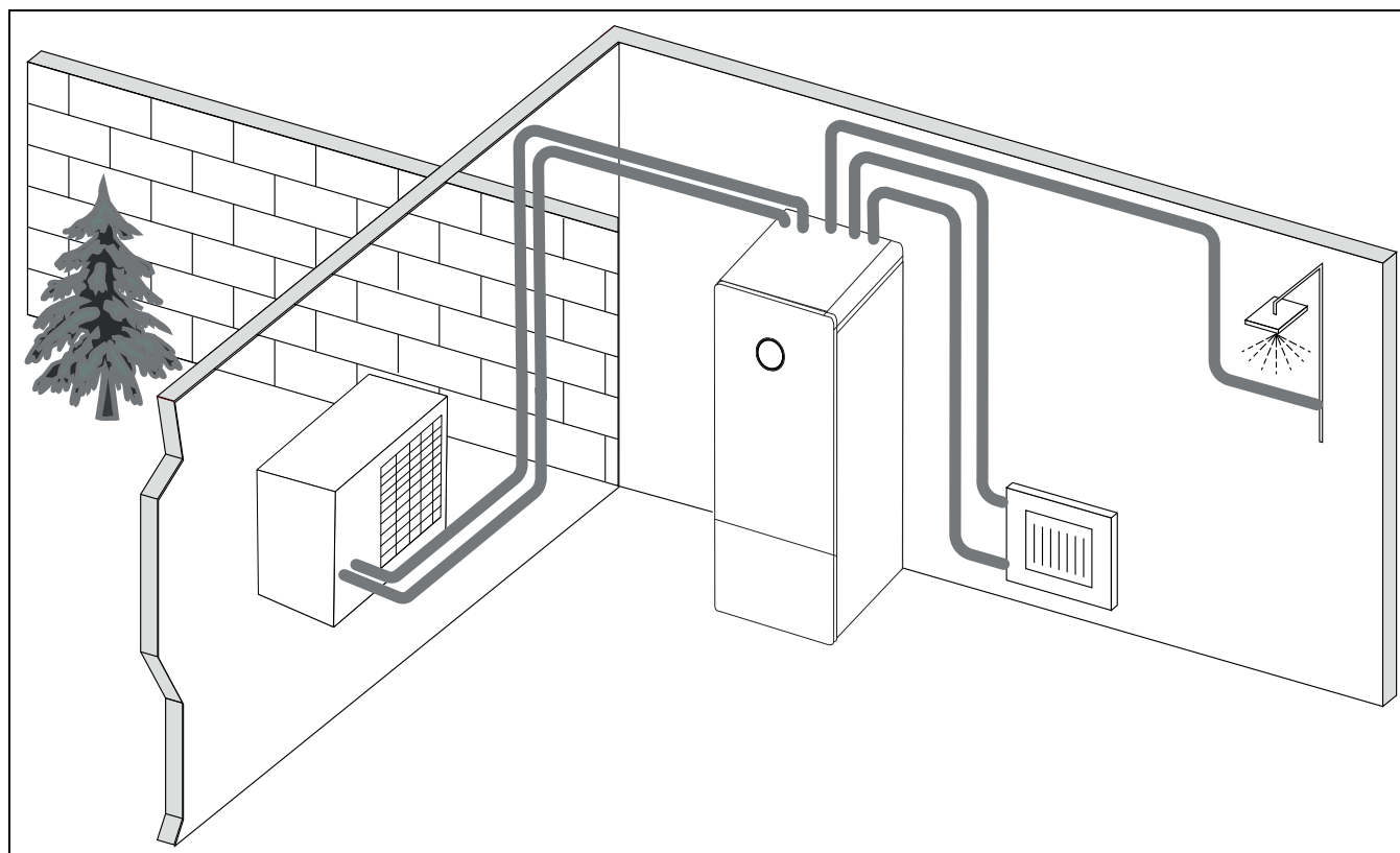
7. ábra AW OR, hőszivattyú, Compress 5800i 12 M beltéri egység beépített használati melegvíz-tárolóval és merülőfűtéssel
