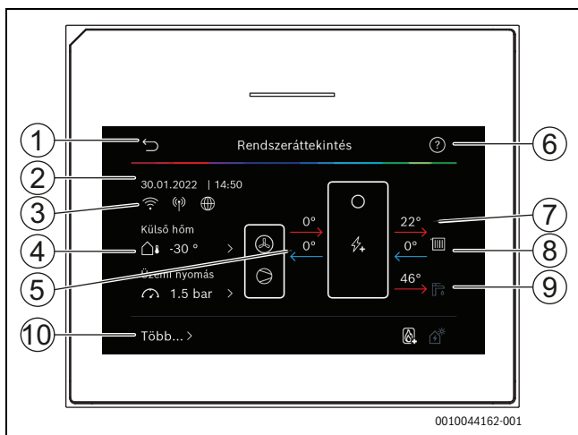
12. ábra Rendszeráttekintés
